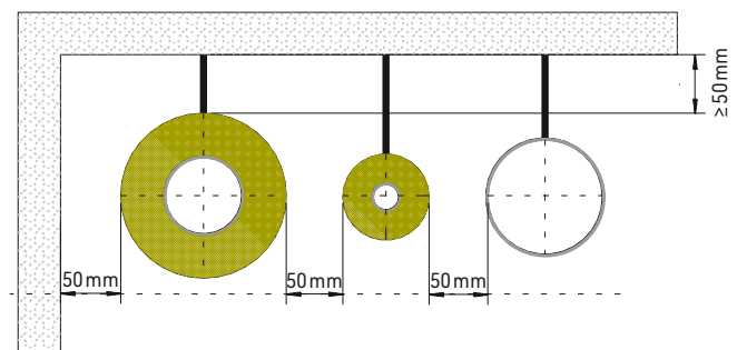
[ABB. 3] Minimalabstände zwischen gedämmten und nicht gedämmten Rohrleitungen.
