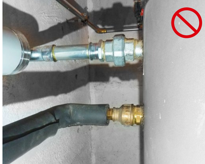
[ABB. 31] Diese Installation zeigt mehrere Nachlässigkeiten gleichzeitig auf: Die Anschlüsse am Warmwasserspeicher sind nicht gedämmt. Die Dämmstärke des synthetischen Kautschuks entspricht nicht den Vorschriften. Die Naht ist nicht richtig verschlossen und sie sollte nicht seitlich, sondern zur Verhinderung der natürlichen Konvektion bevorzugt im unteren Bereich angeordnet sein. An diese Rohrleitung gehört eine klassische Dämmung mit Mineralwolle gemäss kantonalen Energiegesetzen!
