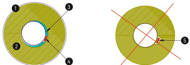
[ABB. 27] Dämmung über Begleitheizung dimensionieren. 1 Umhüllung 2 Dämmstoff 3 Eingeschlossene Luft 4 Elektrische Begleitheizung 5 Auskerbung der Dämmung
