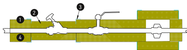
[ABB. 11] Dämmung von Kleinventilen und Rohrverschraubungen.
