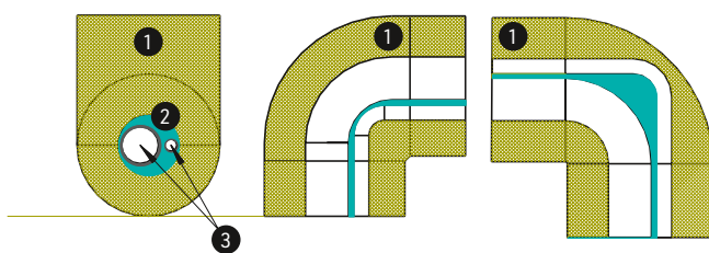
[ABB. 26] «Rohr an Rohr»-Dämmung. 1 Dämmung 2 Eingeschlossene Luft 3 Rohr an Rohr
