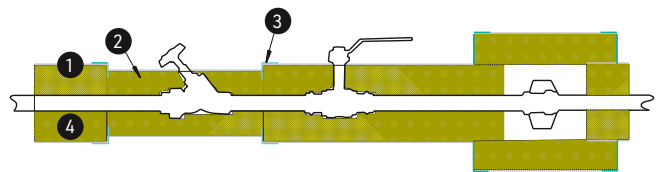
[ABB. 11] Dämmung von Kleinventilen und Rohrverschraubungen.
