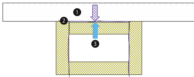
[ABB. 16] Kondensatansammlung zwischen feuchter Betondecke und Dämmung wegen Taupunktunterschreitung infolge von fehlendem Luftaustausch zwischen Decke und gedämmter Lüftungsleitung.
