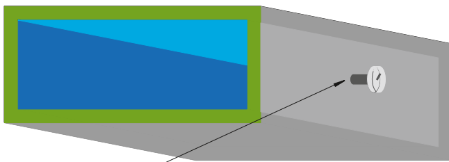
Dämmung von Fühler- und Thermometerstutzen im Tauwasserbereich mit synth. Kautschuk von mind. 13 mm Dicke.
