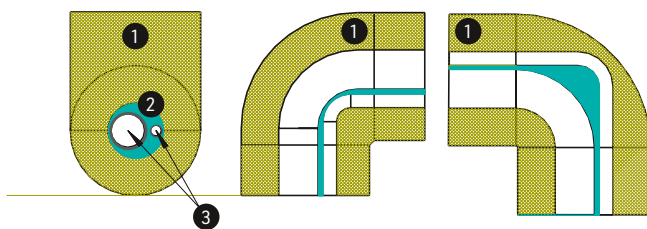
[ABB. 26] «Rohr an Rohr»-Dämmung.
