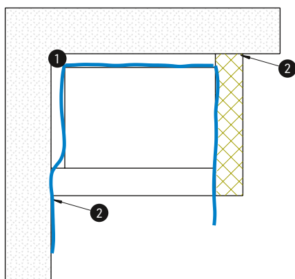
[ABB. 15] Beispiel einer Kondensatansammlung infolge Taupunktunterschreitung nicht gedämmter Lüftungsleitungen.
