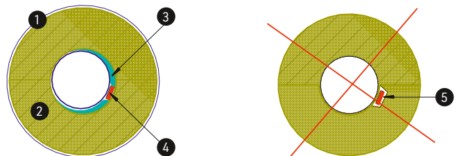
[ABB. 27] Dämmung über Begleitheizung dimensionieren.
