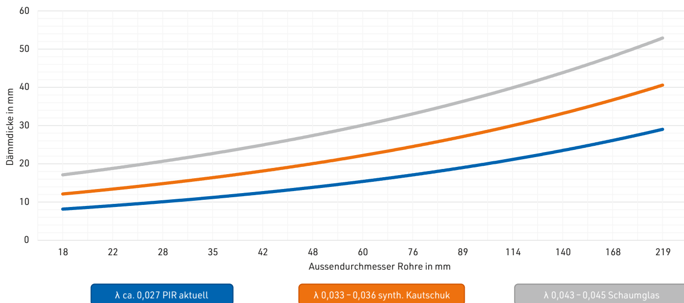
[ABB. 20] Empfohlene Dämmdicken nach Temperatur und \lambda -Wert.
