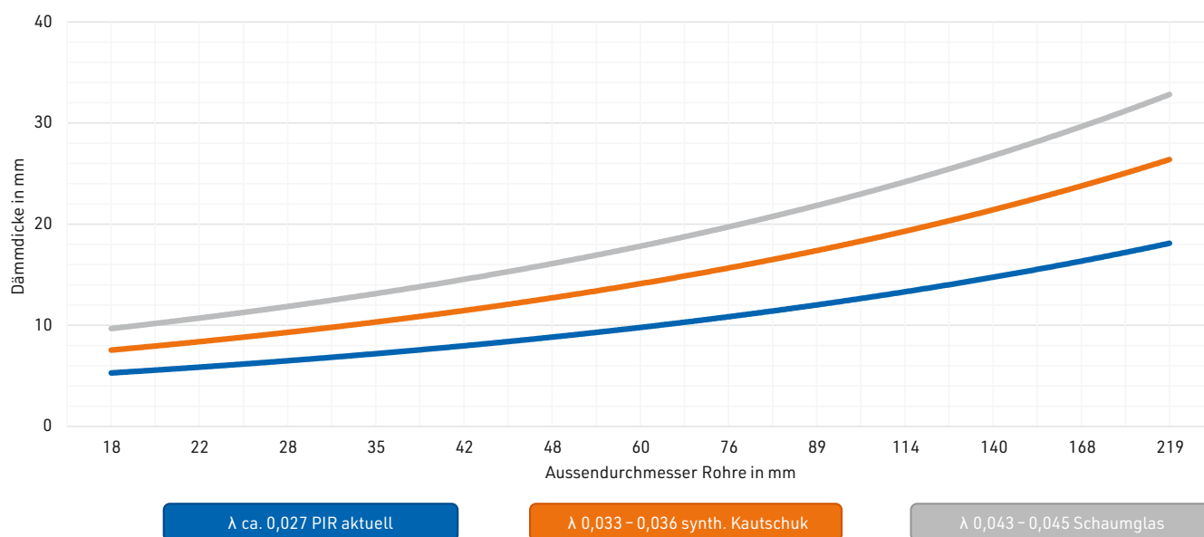
[ABB. 21] Empfohlene Dämmdicken nach Temperatur und \lambda -Wert.
