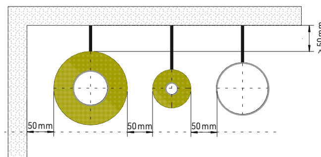
[ABB. 3] Minimalabstände zwischen gedämmten und nicht gedämmten Rohrleitungen.
