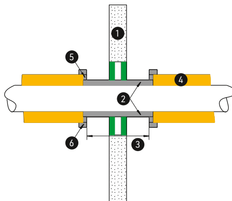
[ABB. 30] Mögliche Ausführung von Brandabschnittsdurchführungen.
