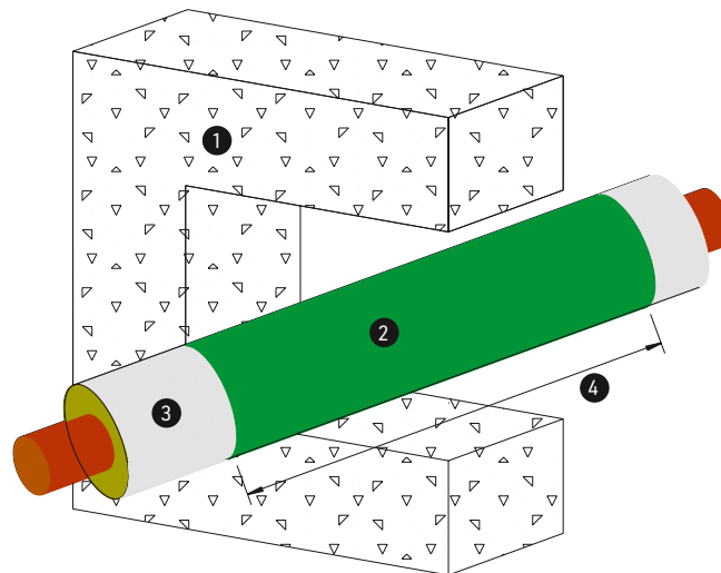
[ABB. 13] Möglicher Dämmaufbau im Bereich des Brandabschnitts.
