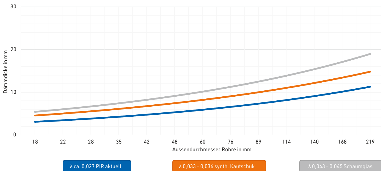
[ABB. 22] Empfohlene Dämmdicken nach Temperatur und \lambda -Wert.
