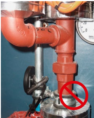
[ABB. 37] Auch schwierige Stellen dämmen!
