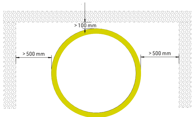
[ABB. 6] Mindestabstand zwischen gedämmtem Behälter und Bauteil oder anderen Installationen.
