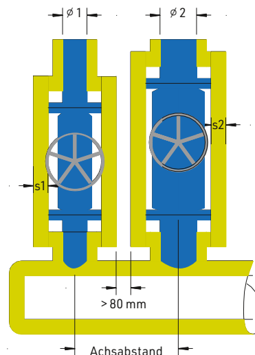
[ABB. 3] Minimalabstände zwischen gedämmten und nicht gedämmten Rohrleitungen.
