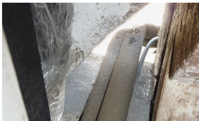
[ABB. 42] In unbeheizten Räumen sind Rohrleitungen gemäss den kantonalen Energiegesetzen zu dämmen. Sie sind gegen UV-Strahlung und weitere Witterungseinflüsse zu schützen.
