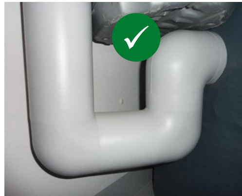
[ABB. 38] Korrekt gedämmter Siphon.
