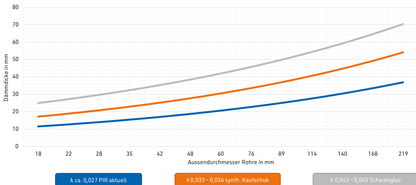
[ABB. 19] Empfohlene Dämmdicken nach Temperatur und \lambda -Wert.
