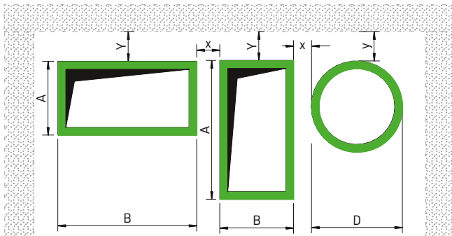
[ABB. 5] Mindestabstand zwischen gedämmten Leitungen zueinander und zum Bauteil sowie zu anderen Installationen.
