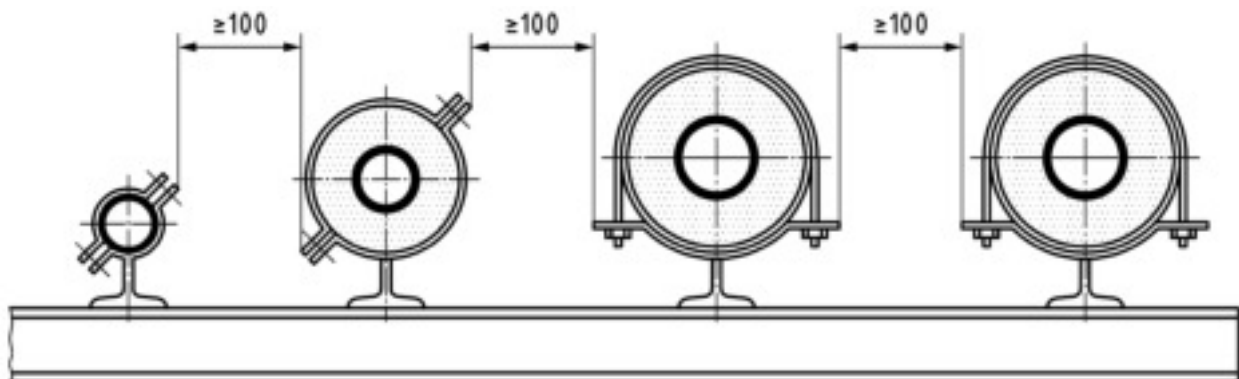
Mindestabstände zwischen gedämmten und ungedämmten Rohrleitungen
